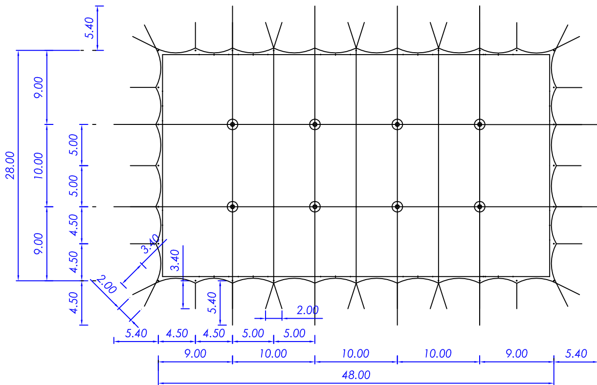
PIANTA COPERTURA
