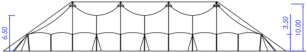
PROSPETTI
